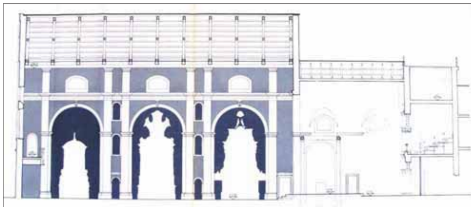
Uzdružni presjek unutrašnjosti crkve, Bernardo Bernardi, 1974. (AFSS, Fond nacrt)
