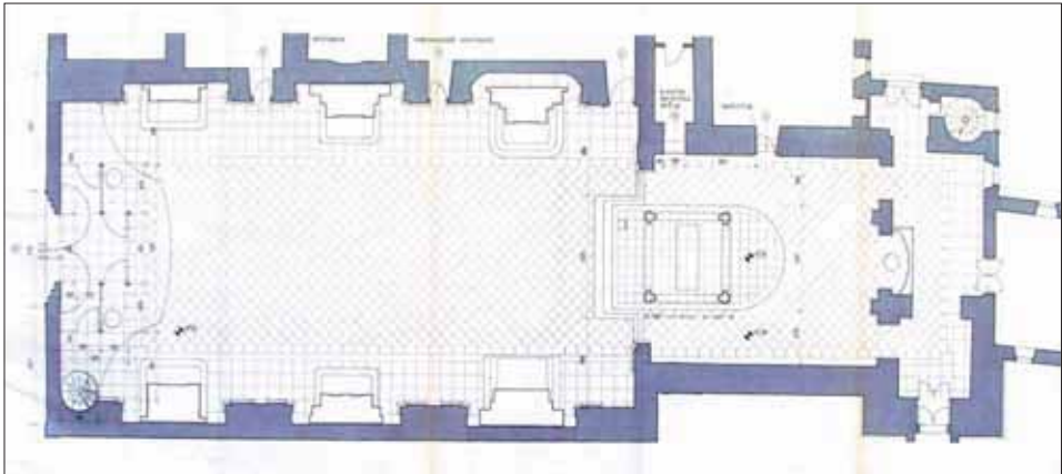
Tlocrt crkve, Bernardo Bernardi, 1974. (AFSS, Fond nacrtu)
