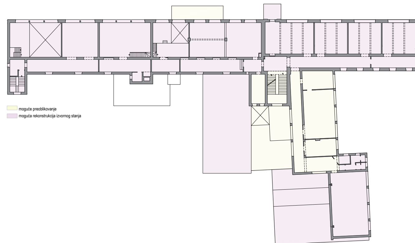
DRUGI KAT
