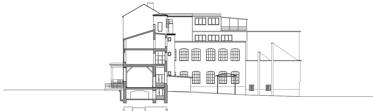
Presjek kroz Grossovu zgradu s pogledom na istok
