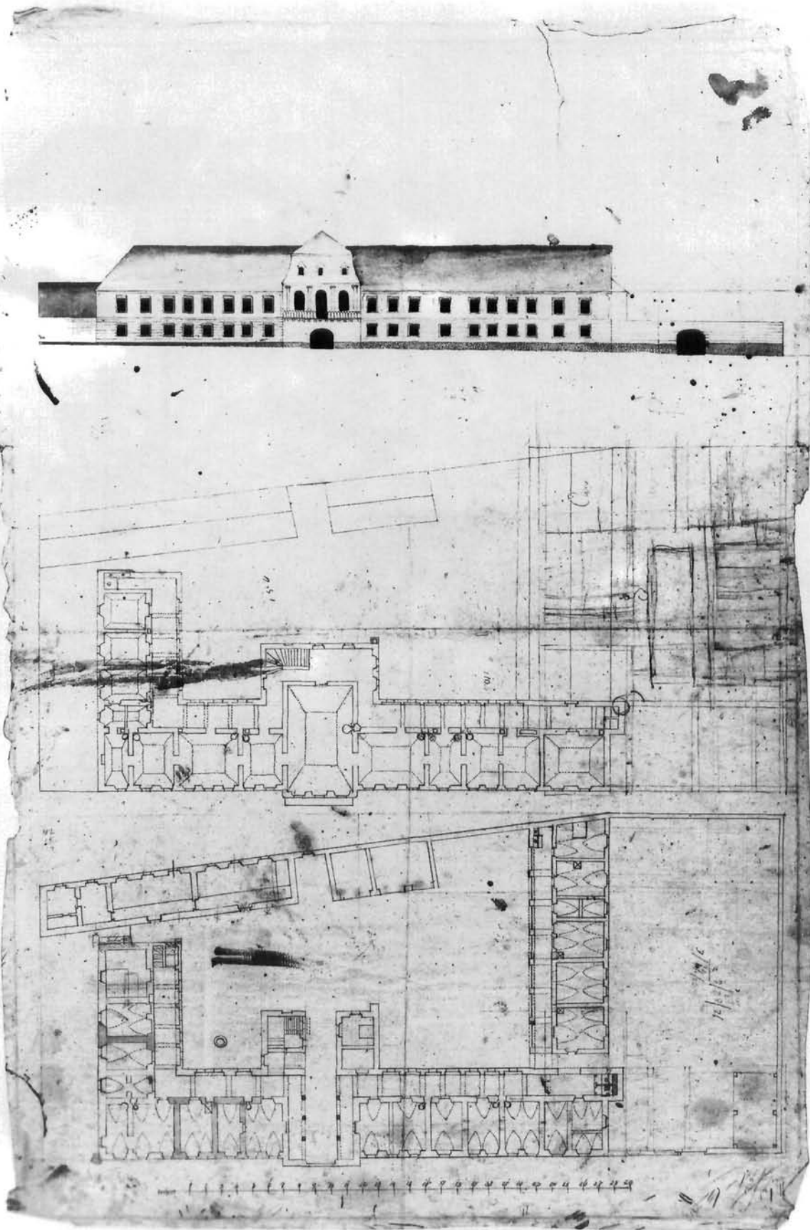
Preris nacрта županijske palače iz 1779/80, Arhiv Hrvatske Copy of plans of district palace (1779/80, Archives of Croatia)
