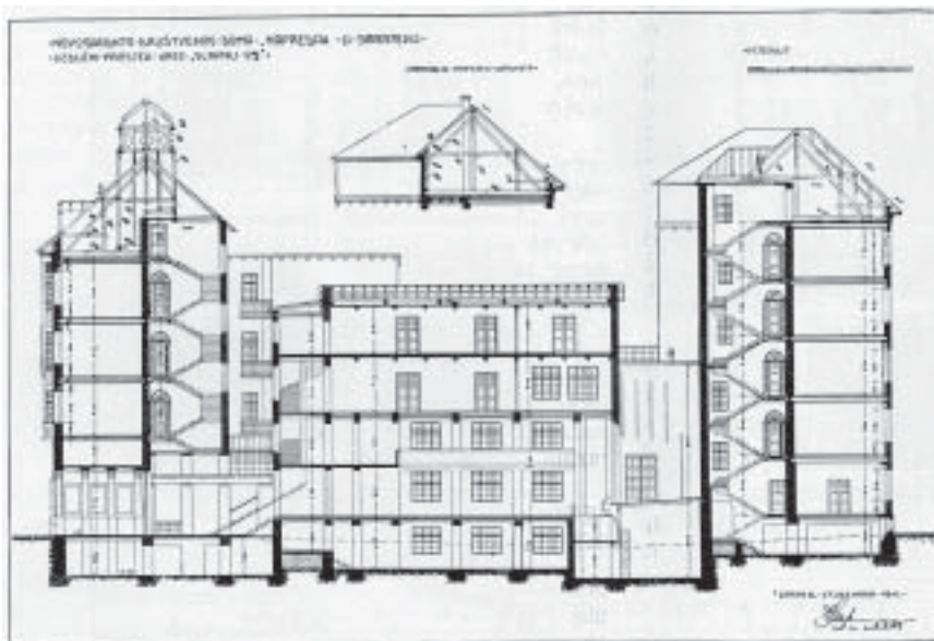
D. Sunko, Napretkov zakladni dom , Sarajevo, uzdužni presjek kroz glavnu os, studeni 1911. (»Viesti Hrvatskog društva inžinira i arhitekata«, 1913.)
