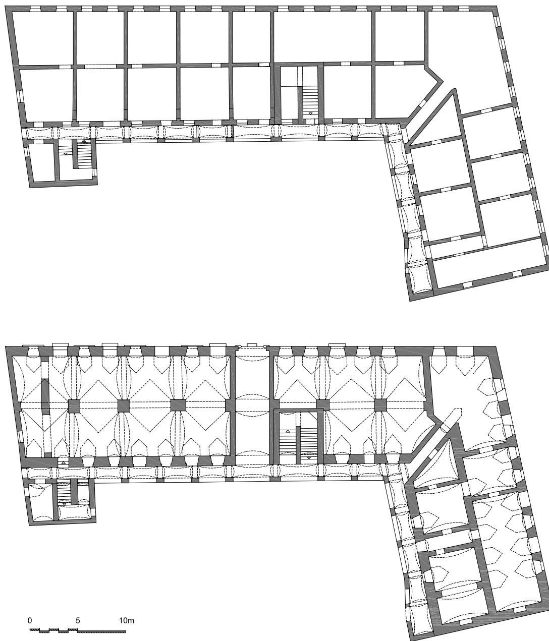
9. Palača Pejačević, tlocrt kata i prizemlja, rekonstrukcija II. faze izgradnje (arhitektonska snimka: Atelier X, grafička obrada Ivana Valjato-Vrus) Pejačević Palace, ground plan of the upper and ground level, reconstruction of the 2 nd building phase
