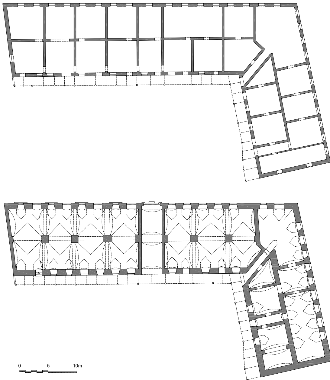
6. Palača Pejačević, tlocrt kata i prizemlja, rekonstrukcija I. faze izgradnje (arhitektonska snimka: Atelier X, grafička obrada Ivana Valjato-Vrus).
