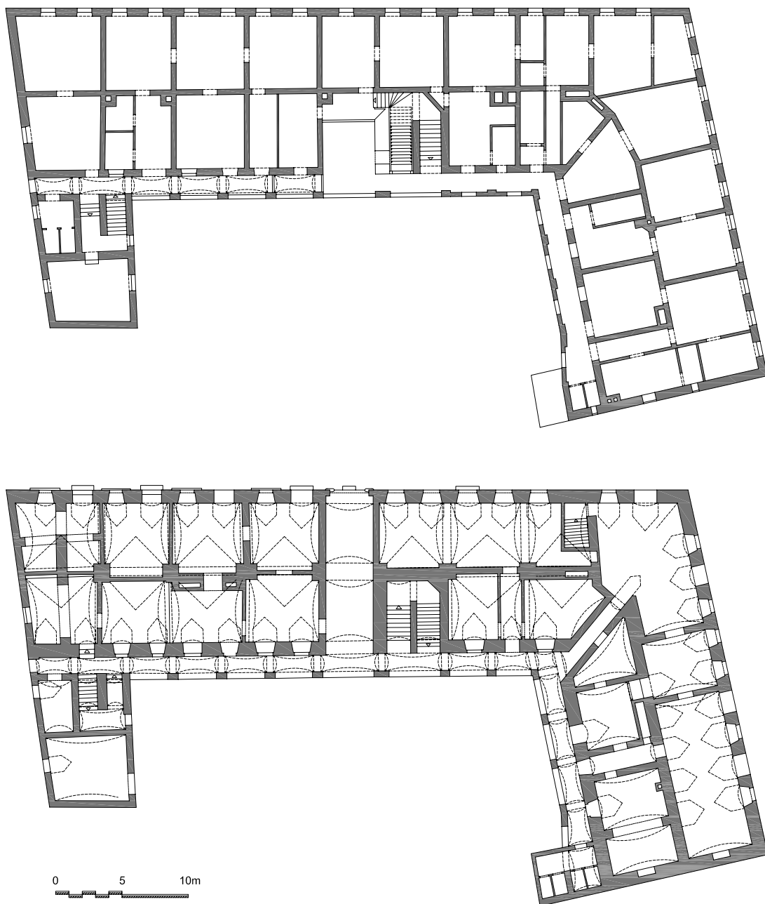
2. Palača Pejačević, tlocrt prizemlja i kata, postojeće stanje (arhitektonska snimka: Atelier X, grafička obrada Ivana Valjato-Vrus)
