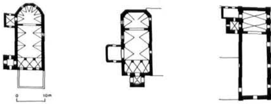
Močila, crkva B. D. Marije, poč. 18. stoljeća, tlocrt
