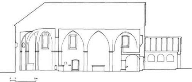
Močila, crkva B. D. Marije, uzdužni presjek
